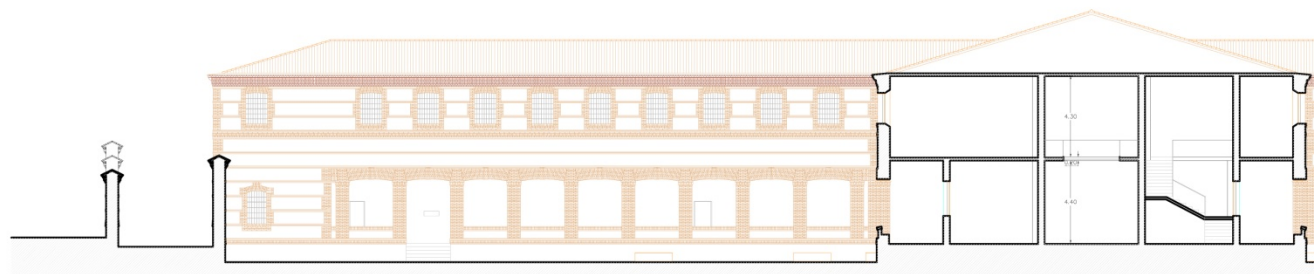
ALZADO-SECCIÓN SUR 2
